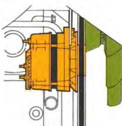
Växelströmgenerator ger laddning redan vid låga varvtal.
