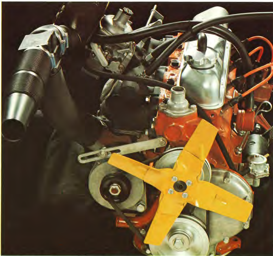
Ny 2 liters B 20-motor med speciellt goda lågvarvsprestanda. 90 alt. 118 hk SAE.
