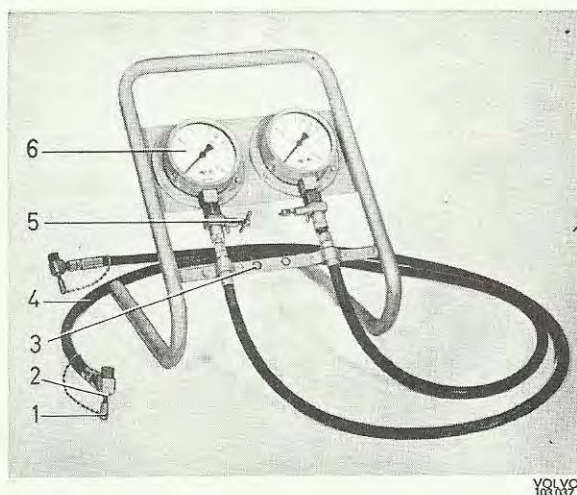
Bromstrycksmätare 999 2741
