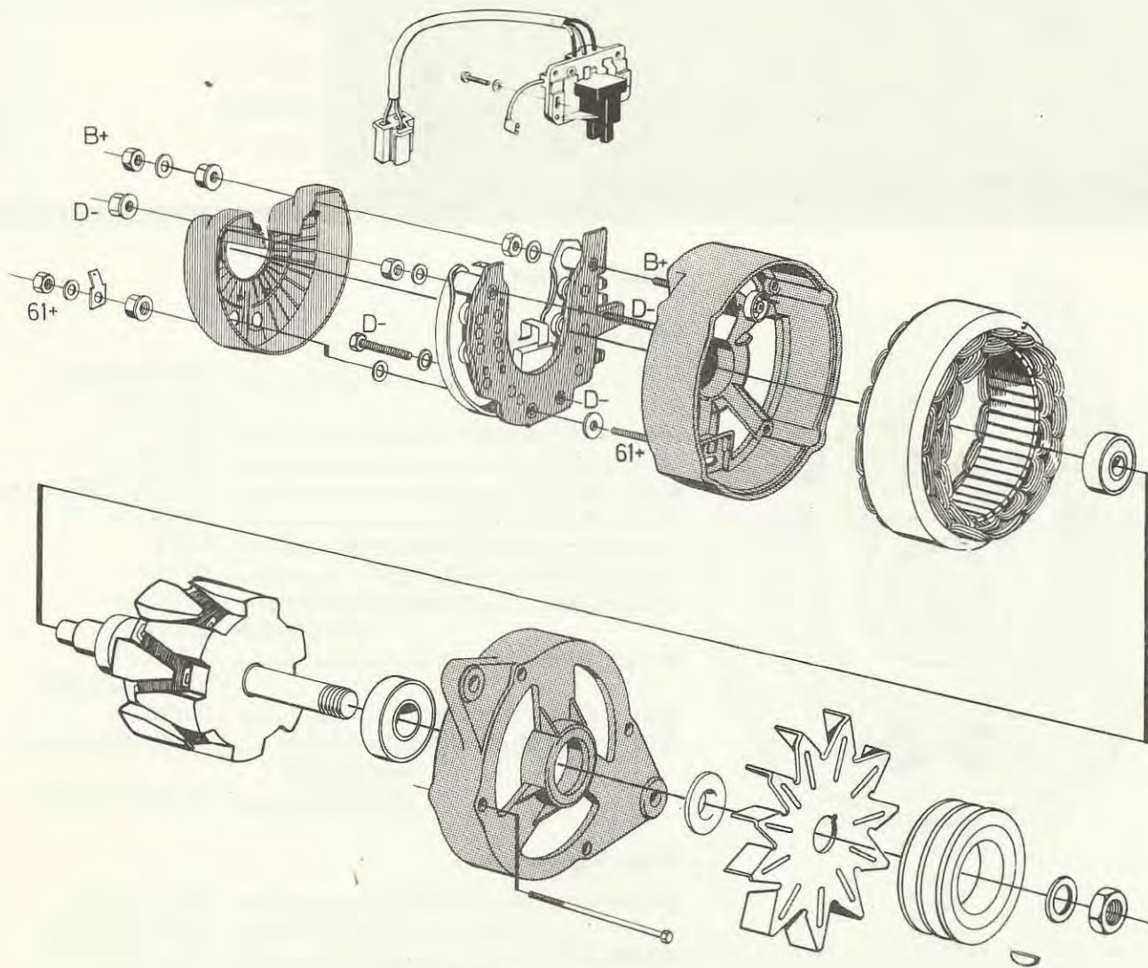
Sprängbild 70 A Generator
