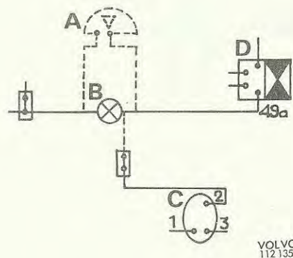
Kopplingschema
