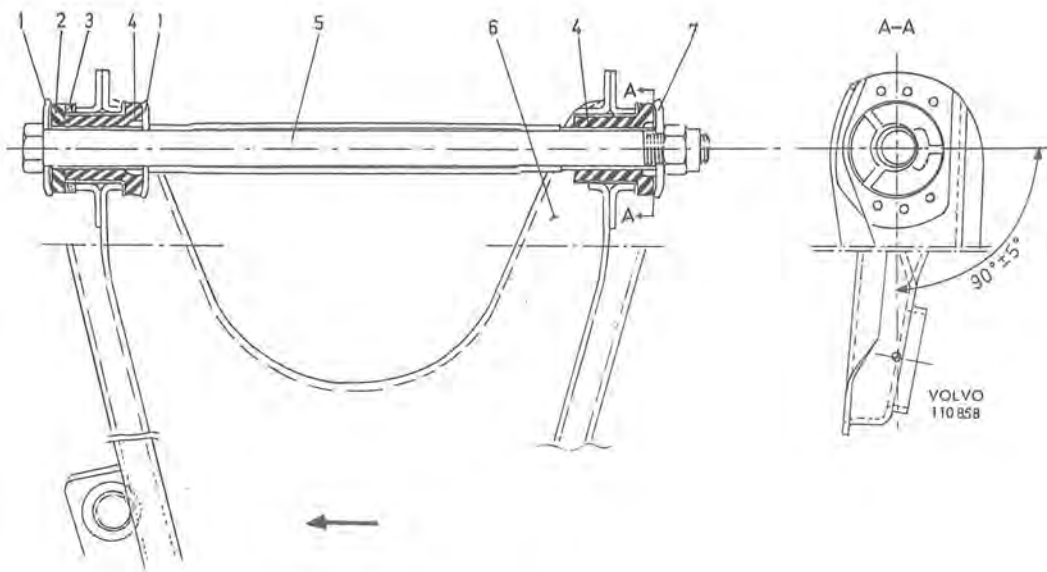
Nedre länkarm
