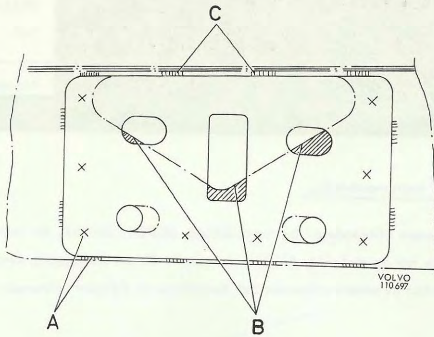
Bild 2 Täckplätens fastsättning
