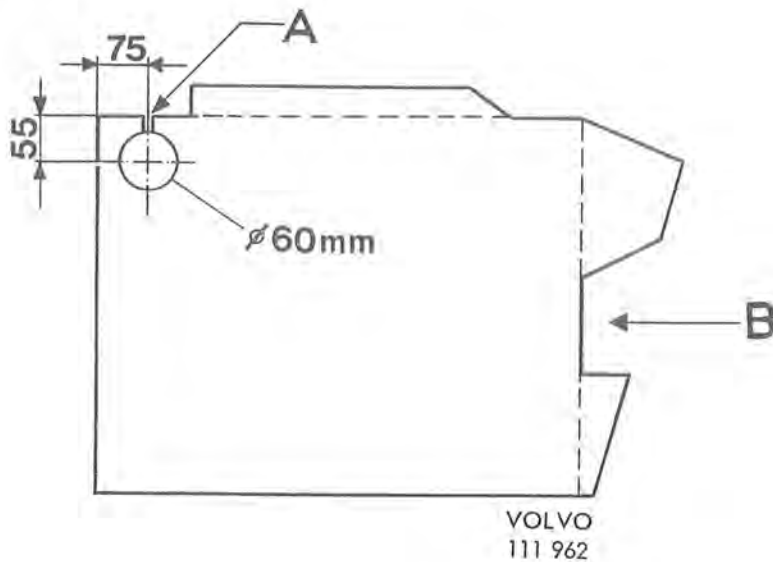
Bild 2. Håltagning i ljudvall
