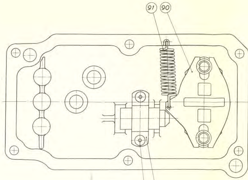
VY F-F
