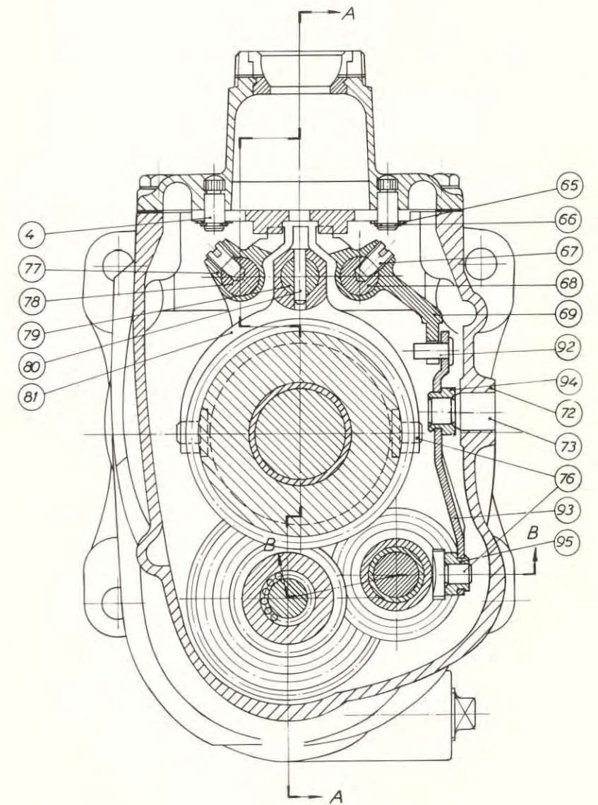
SNITTE-E
