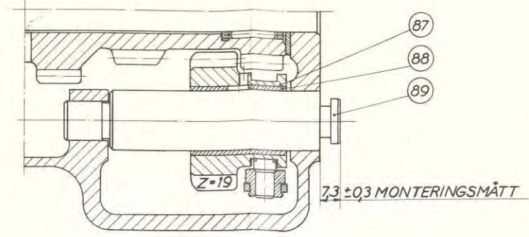
SNITT B-B
