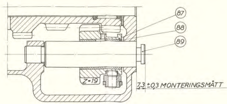
SNITT B-B
