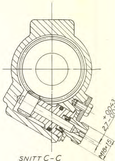
SNITT C-C
