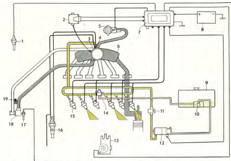
Principbild bränslesystem B 30 E
