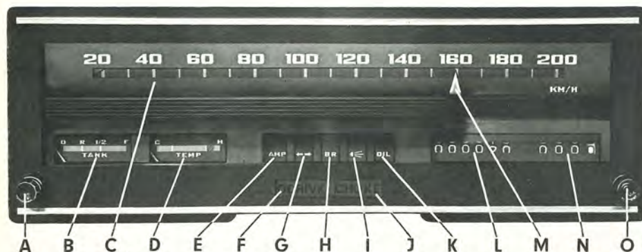
D Temperaturmätare, kylvätska
