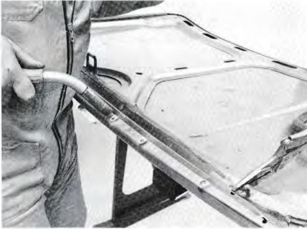
Punktsvetsa plåtarna.
