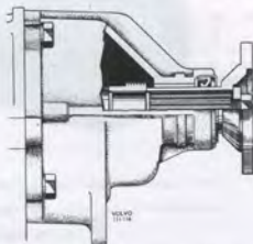
Bild 4. Bakre hus, automatväxellåda
