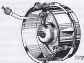
Bild 2. Hållare för strålkastarinsats
