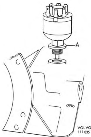
Bild 1. Montering av startspärrkontakt
