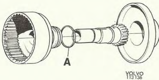
A. Tätningring
