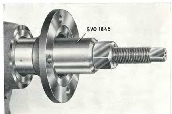
Bild 5. Montering av medbringare
