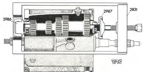
Bild 26. Montering av främre innerring
