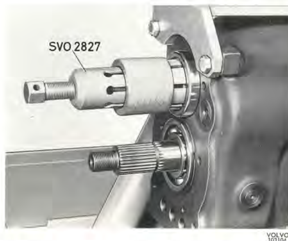
Bild 10. Demontering av mellanaxelns bakre lager
