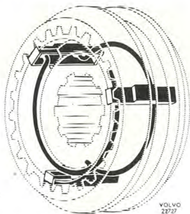
Bild 20. Hopsättning av synkronisering
