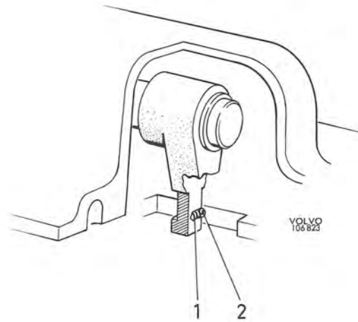
Bild 28. Dämpkula i växelförare
