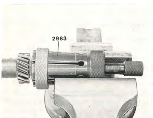
Bild 16. Demontering av bakre innerring
