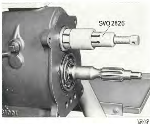
Bild 9. Demontering av mellanaxelns främre lager
