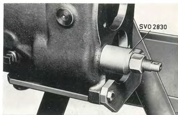
Bild 17. Demontering av backaxel
