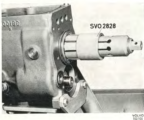
Bild 12. Demontering av huvudaxelns bakre lager M 400
