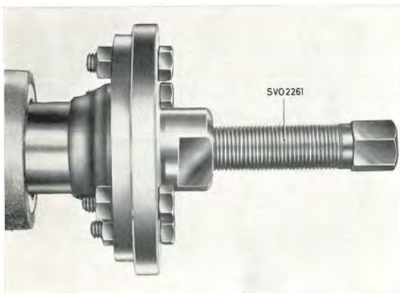
Bild 4. Demontering av medbringare
