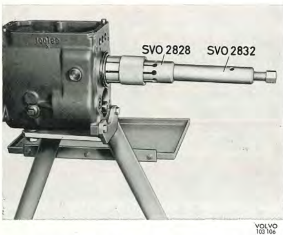
Bild 13. Demontering av huvudaxelns bakre lager M 410
