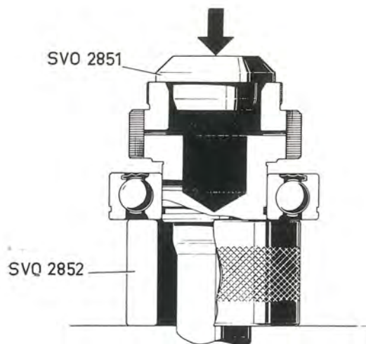
Bild 23. Montering av kullager på ingående axel
