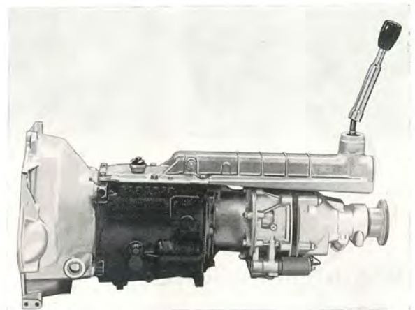
Bild 3. Växellåda M 410
