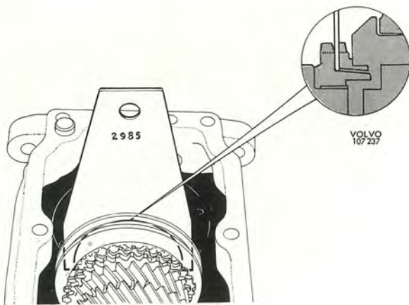
Bild 11. Mothåll för huvudaxel
