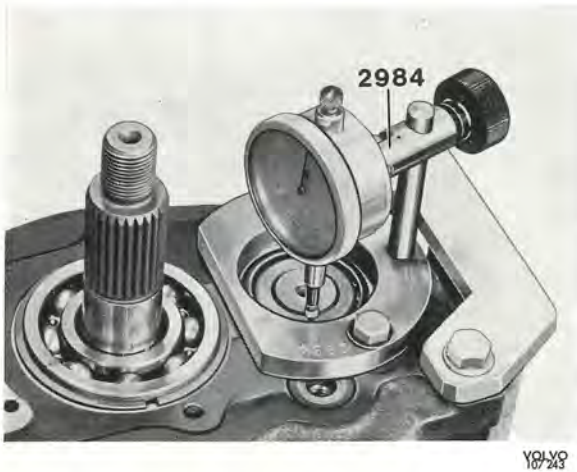
Bild 27. Mätning av axialspelet
