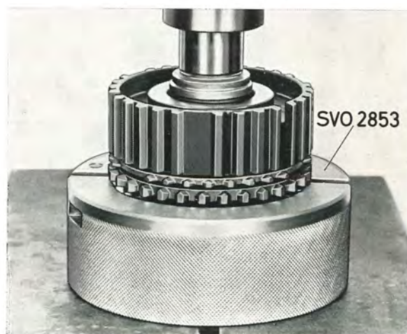
Bild 19. Isärtagning av huvudaxel, II
