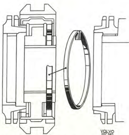
Bild 21. Montering av bromsfjäderring
