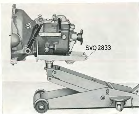
Bild 7. Fixtur för demontering av växellåda
