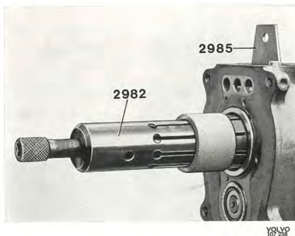
Bild 14. Demontering av lager för ingående axel
