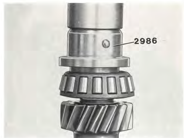
Bild 24. Montering av bakre innerring
