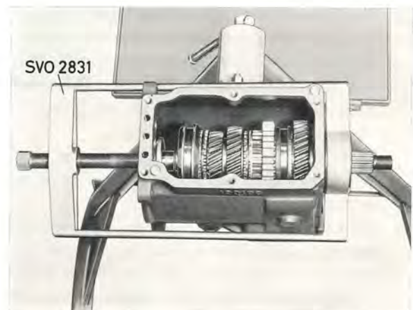
Bild 25. Montering av huvudaxelns bakre lager
