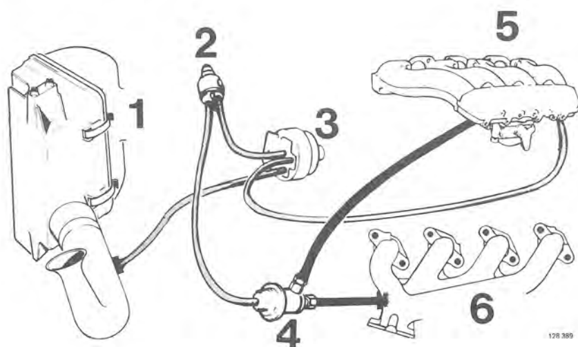
Principskiss (steglöst), tidigt utförande
