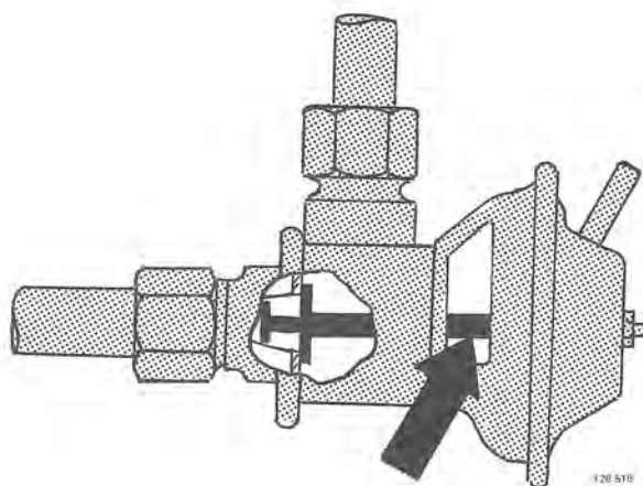
Vakuümventil. Stängd vid kall motor
