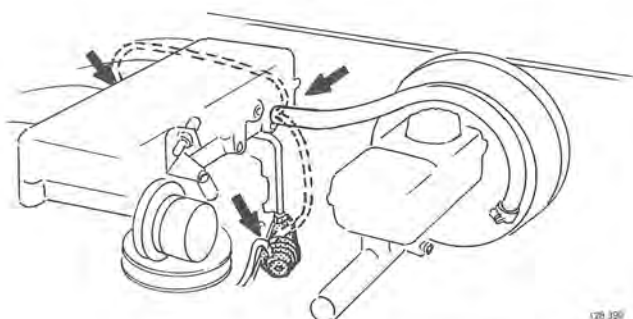
Vakuumventilen. Läge vid varvtal över tomgång med varm motor
