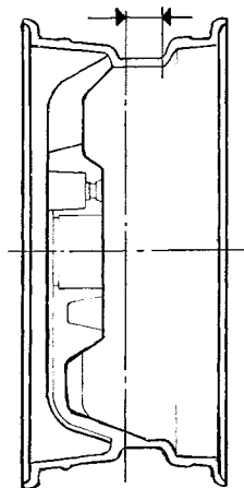
1980 års lättmetallfälg
