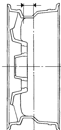
Tidigare lättmetallfälg
