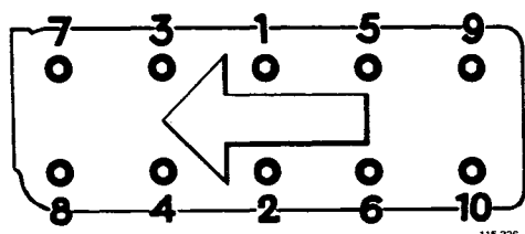
Åtdragningsföljd för cylinderhuvudskruvar
