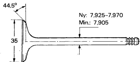
Utloppsventil
