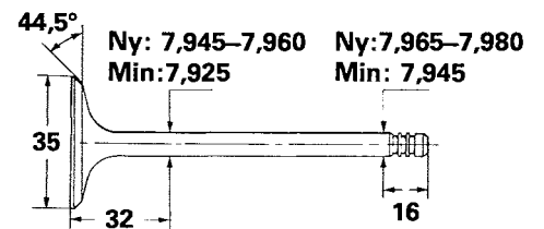
Utloppsventil Turbo-motorer
