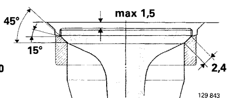
Säte för utloppsventil
