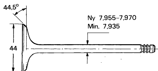
Inloppsventil
