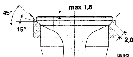
Säte för inloppsventil
