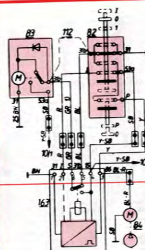
BAKGRÄNSARE, SPOLARE REAR WINDOW WIPER
